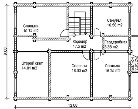
План 2 этажа
