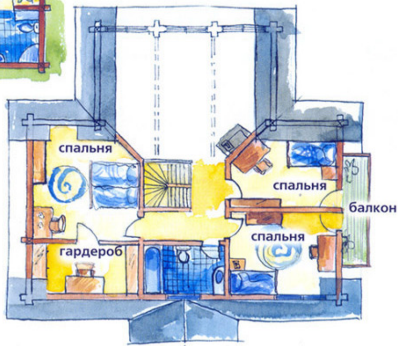
план 2 этажа
