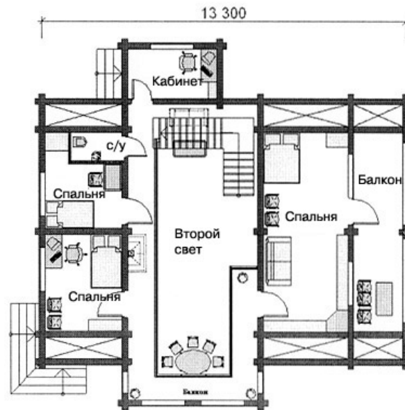
ПЛАН МАНСАРДЫ
